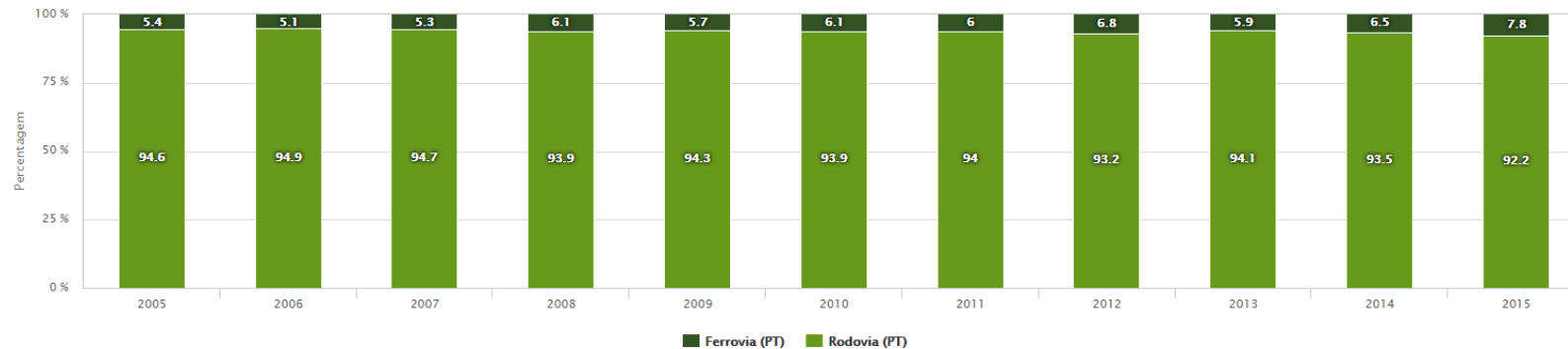
Distribuição modal do transporte de mercadorias, na UE-28
